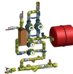
Incluye bomba doble 1º y 2º, interc. de placas, mat. hidráulico y c.e. con centralita
